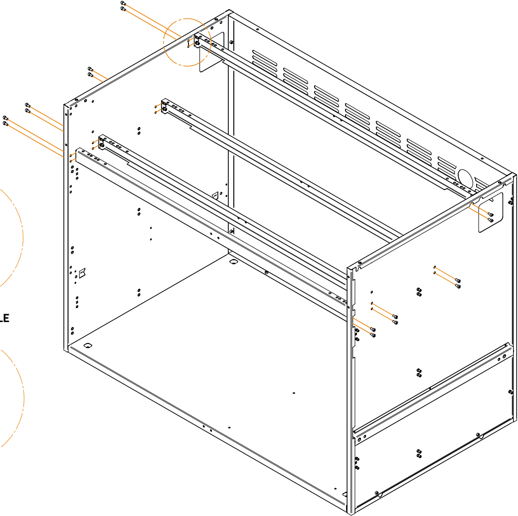
GRILL MODULE
